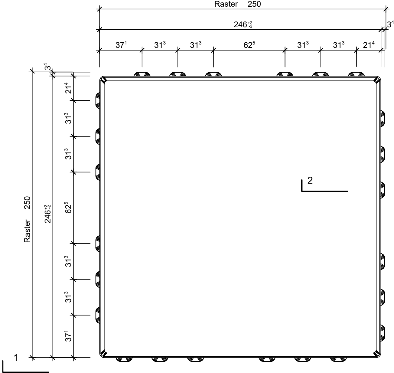
Grundriss 1:2
