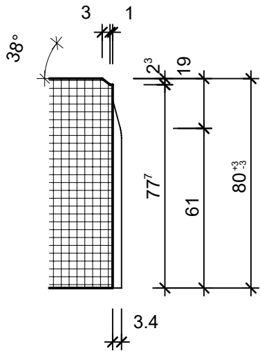
Schnitt 2-2, 1:2
