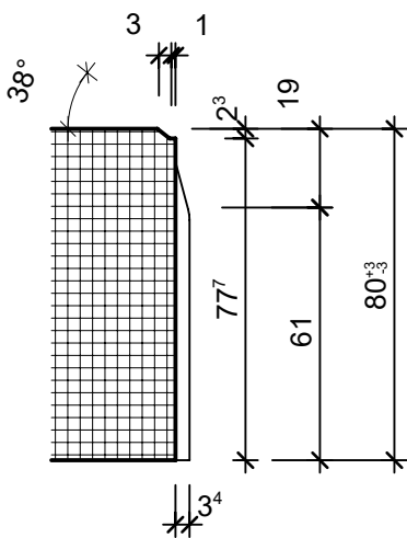
Schnitt 2-2, 1:2
