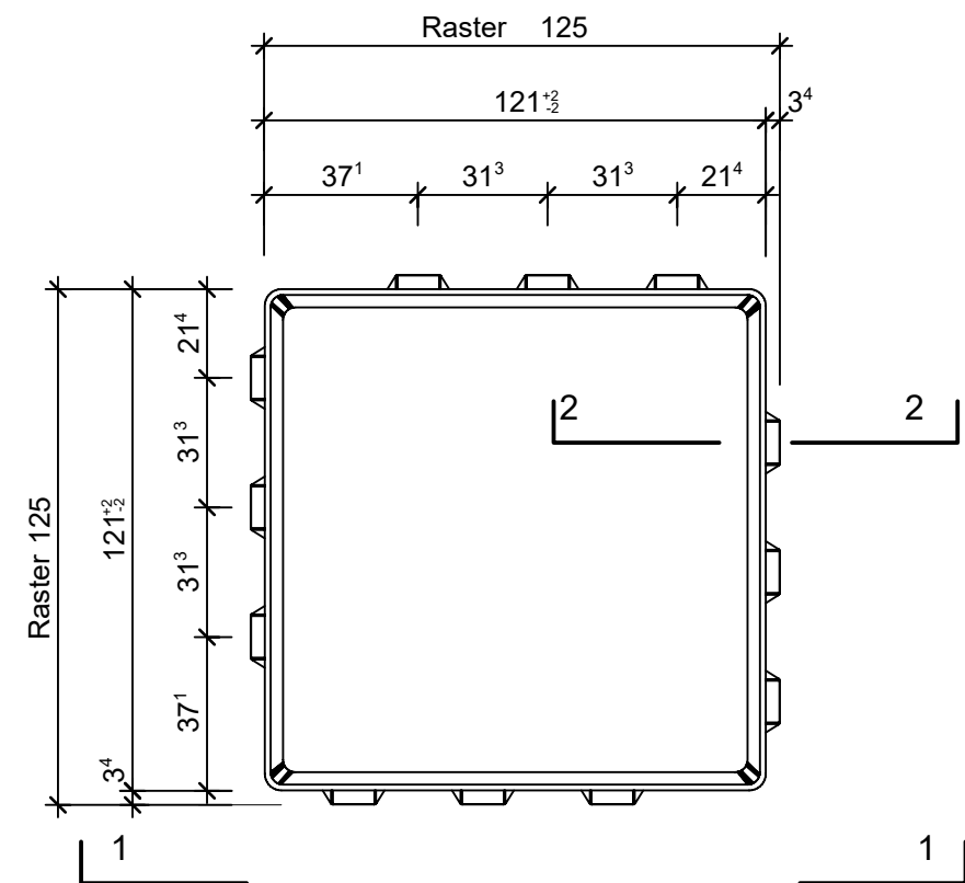
Grundriss 1:2
